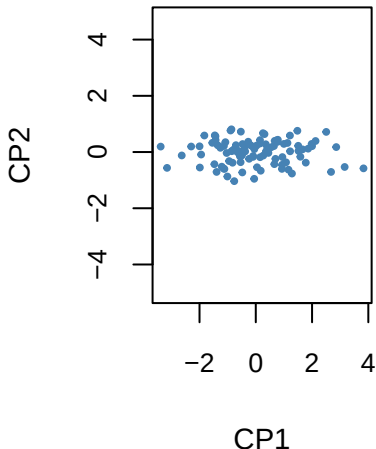
Plano PCA
