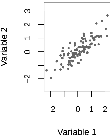
Variables originales
